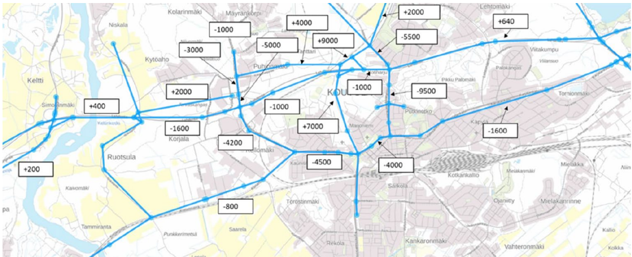
Kuva 32. Ote Vt6 tiesuunnitelmaraportista: Hankkeen aiheuttamat liikenteen siirtymät nykytilanteesta ja vaikutus keskimääräiseen vuorokausiliikenteeseen ajoneuvoa vuorokaudessa (KVL).
