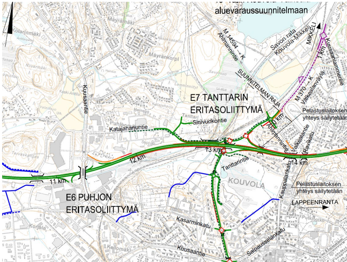
Kuva 27. Ote valtatie 6 yleissuunnitelmasta Tanntarin kohdalla.
