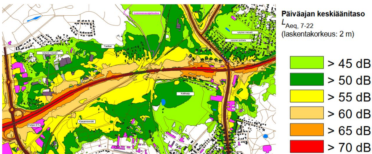
Kuva 16. Ote valtatie 6 tiesuunnitelman meluselvityksestä, melun nykytilanne.
