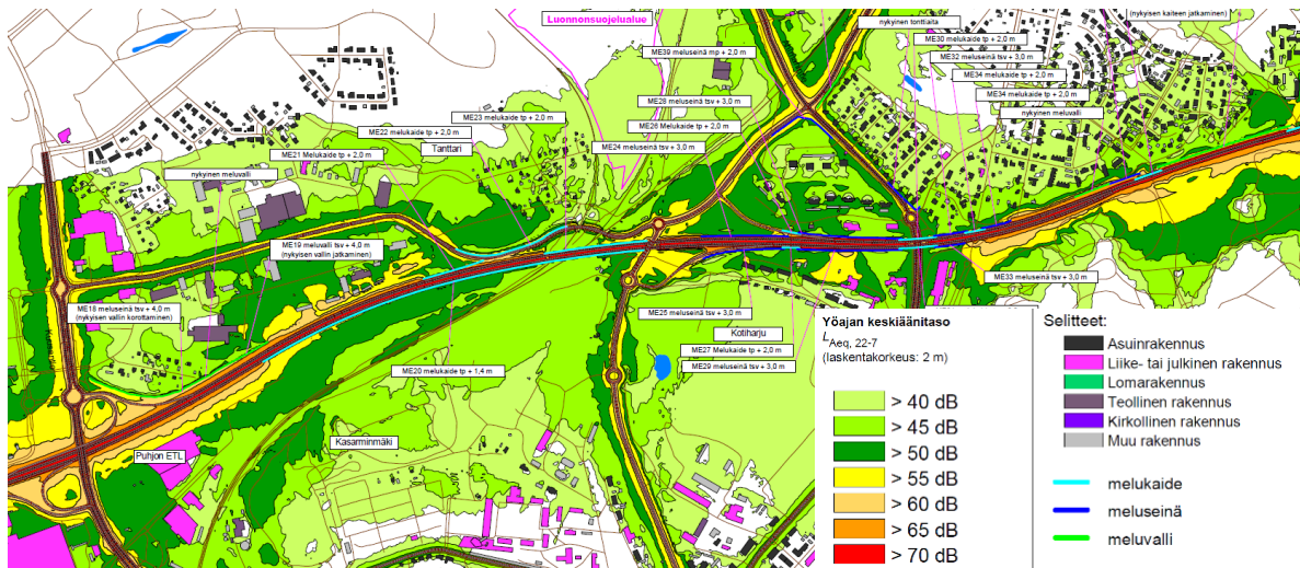
Kuva 33. Ote Vt6 parantamisen Keltti-Tanttari tiesuunnitelman meluselvityksestä. Kuvassa on esitetty meluvyöhykkeet suunnitelluilla väyläratkaisulla ja meluntorjunnalla ennustevuoden 2050 liikennemäärällä.
