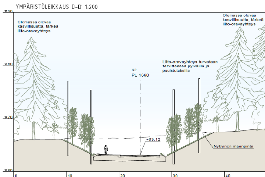
Kuva 40. Esimerkkikuva tiesuunnitelman liito-oravayhteyksien vahvistamisesta Katajaharjuntien kohdalla.
