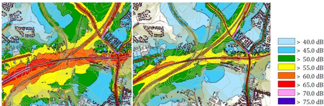
Kuva 15. Otteet Kouvolan kaupungin meluselvityksestä päivä- ja yöajan keskiäänitasoilla.
