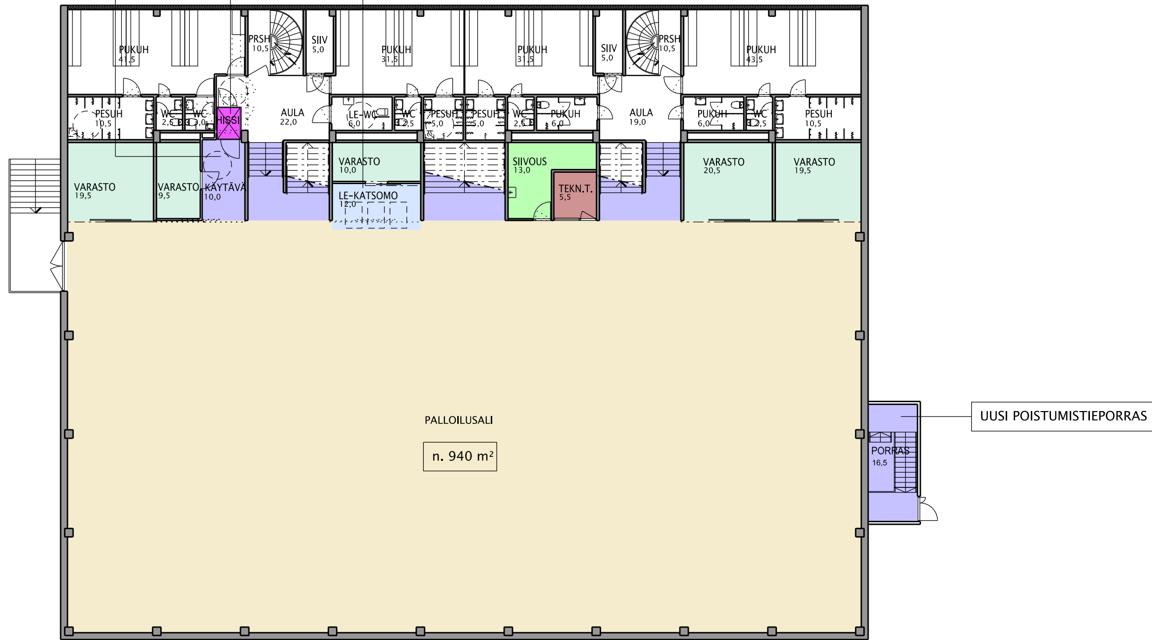
P2 kerros (=PALLOILUSALI +72.623)
