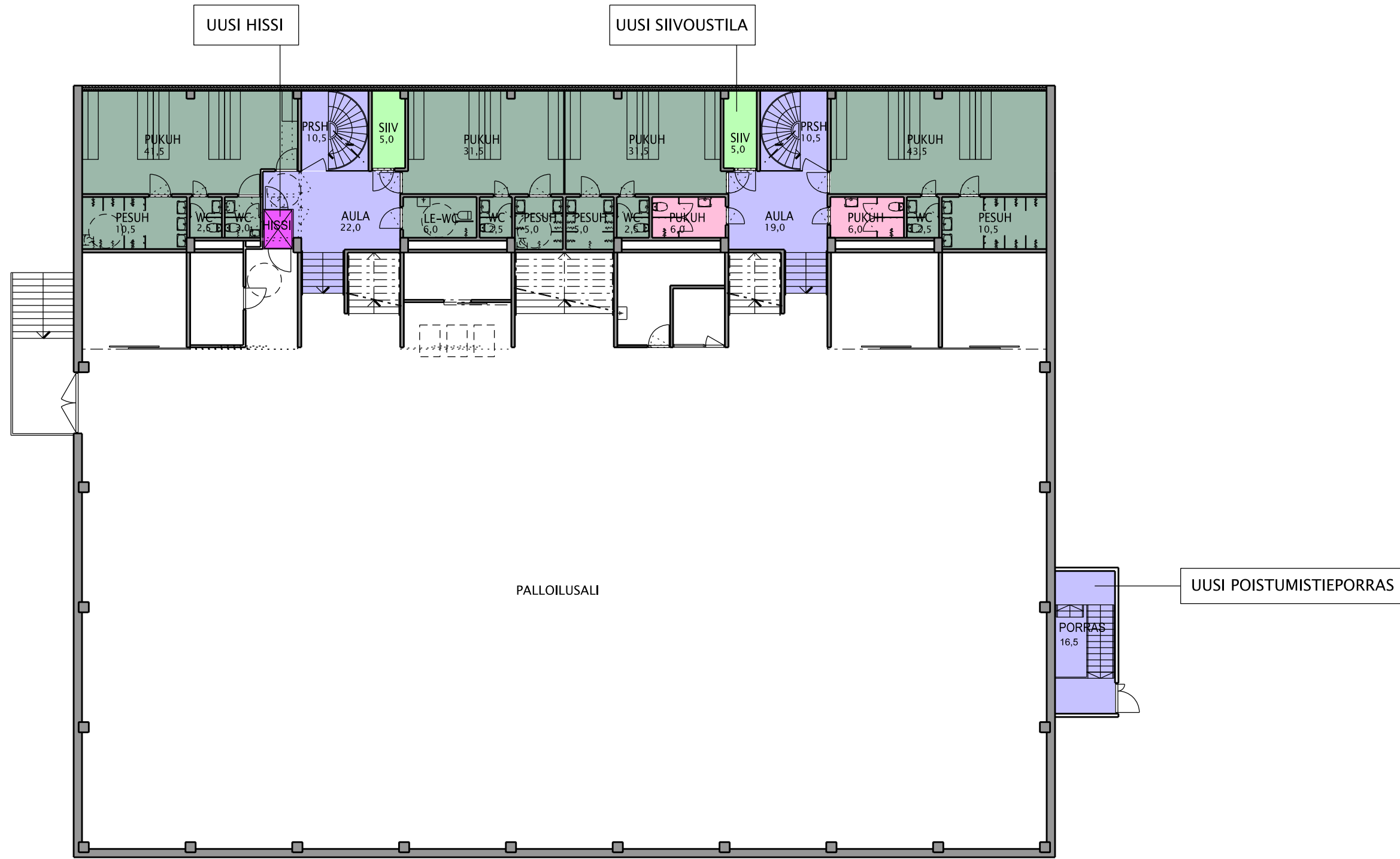
P1 kerros (=PUKUHUONEKERROS +71.523)
