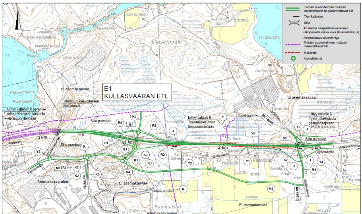
Kuva 28. Ote Vt6 aluevaraussuunnitelmasta Tykkimäki-Häkämäki (SitoWise Oy).
