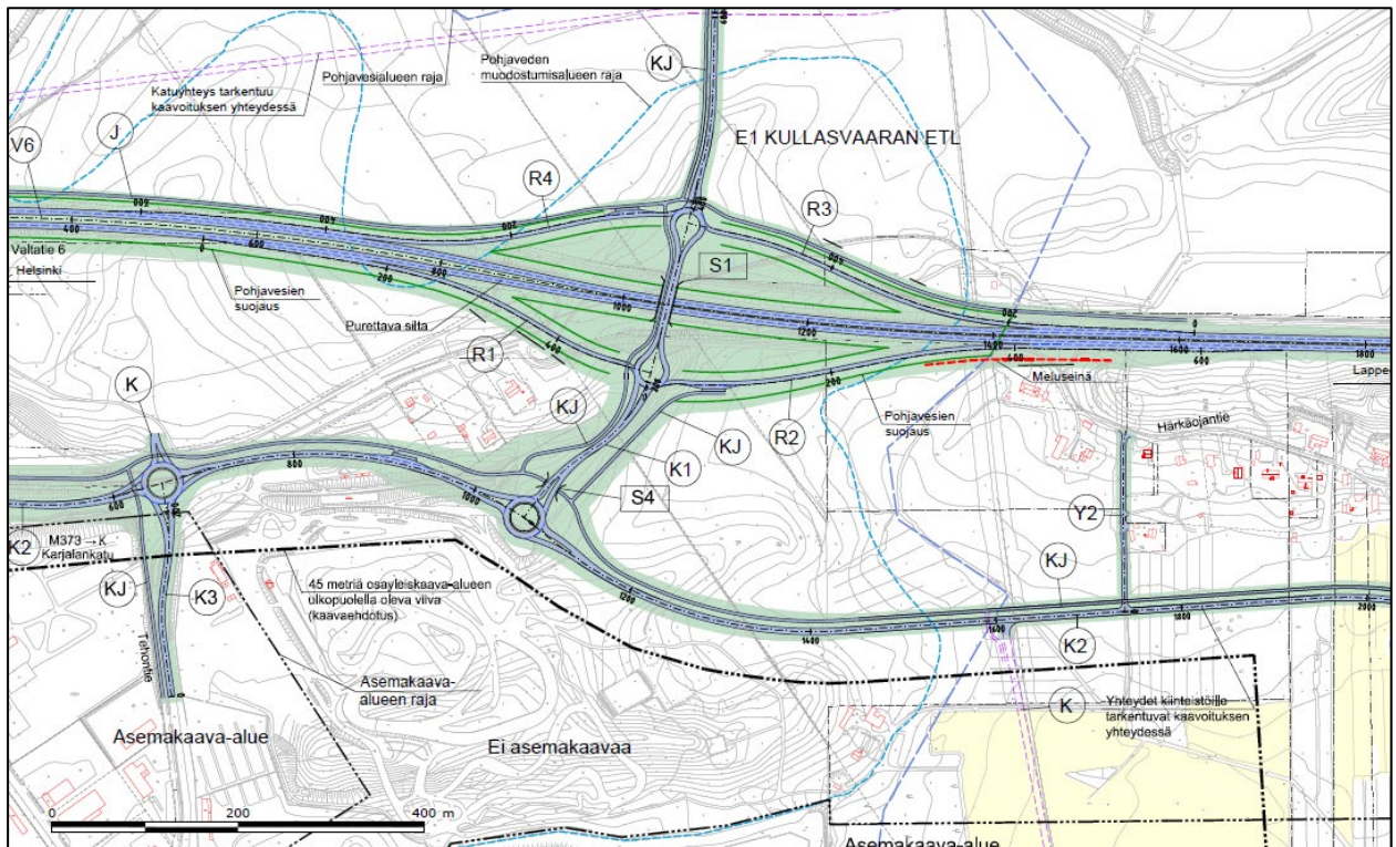
Kuva 27. Ote Vt6 aluevaraussuunnitelmasta Tykkimäki-Häkämäki (SitoWise Oy). Aluevaraussuunnitelma on osa Kullasvaara-Tykkimäki osayleiskaavaa. Eritasoliittymän toteuttaminen vaatii tiesuunnitelman laatimisen.
