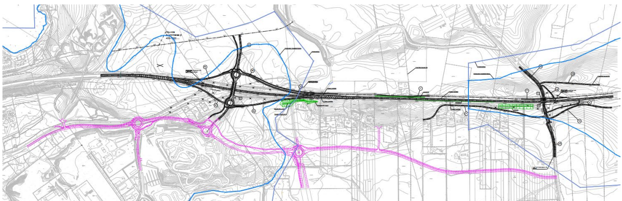
Kuva 33. Tiesuunnitelmaluonnos 4.6.2024.
