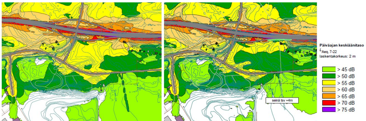
Kuva 43. Otteet valtatie 6 aluevaraussuunnitelman tavoitetilanteen (vuosi 2040) melumallinnuksista (aluevaraussuunnitelman luonnosaineisto). Vasemmassa kuvassa mallinnus ilman meluntorjuntaa ja oikeanpuoleisessa kuvassa mallinnus yleissuunnitelmatasolla mallinnetulla meluntorjunnalla (SitoWise Oy).
