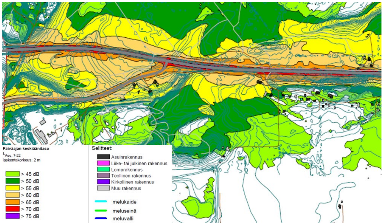
Kuva 21. Ote Vt6 aluevaraussuunnitelman yhteydessä laaditusta Vt6:n nykytilanteen meluvyöhykkeistä päiväaikaan (klo 7-22) (Sito-Wise).
