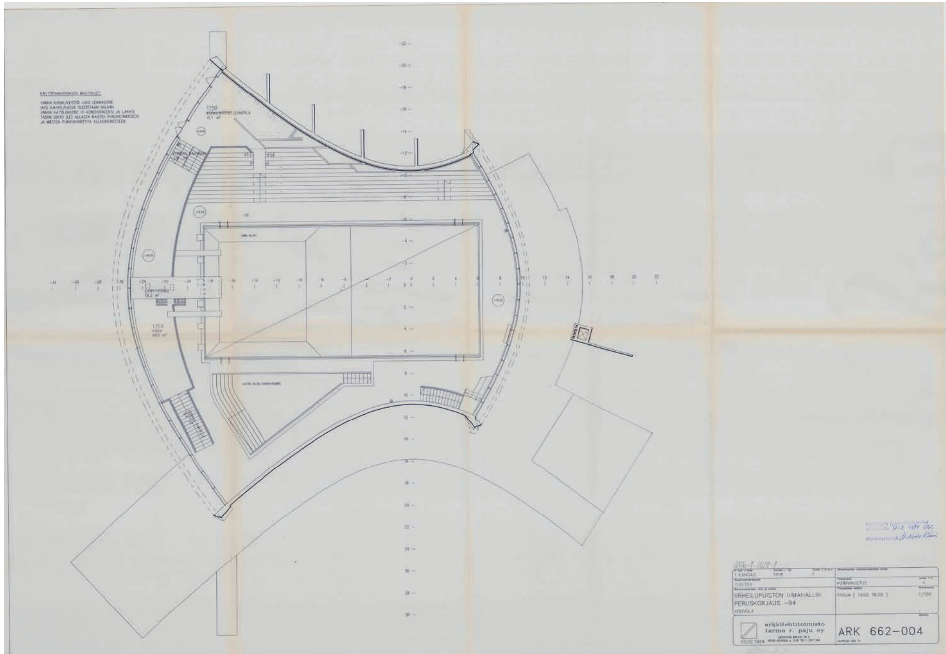
Urheilupuiston uimahallin peruskorjaus 1994. Pohjapiirros, taso +78.05, päiväys 3.2.1994. Pääpiirustukset on hyväksytty 16.2.1994. Kuva: Kouvolan kaupunki, rakennusvalvonnan arkisto.
