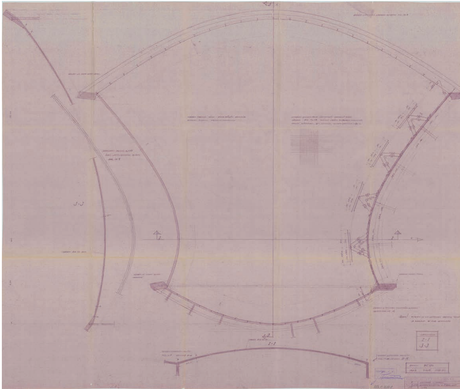
Kouvolan uimahallin kuoren raudoitus ja 1. kerroksen katto, päiväys 13.6.1962. Kuvassa mm. satulakaton (hyperboloidinen paraboloidi) betonikuoren yhdistyminen lapekattoon ja kuorirakenteen paksuuden vaihtelun mitoja. Rakennepiirustusnumero 5. Kuva: Kouvolan kaupunki, rakennusvalvonnan arkisto.
