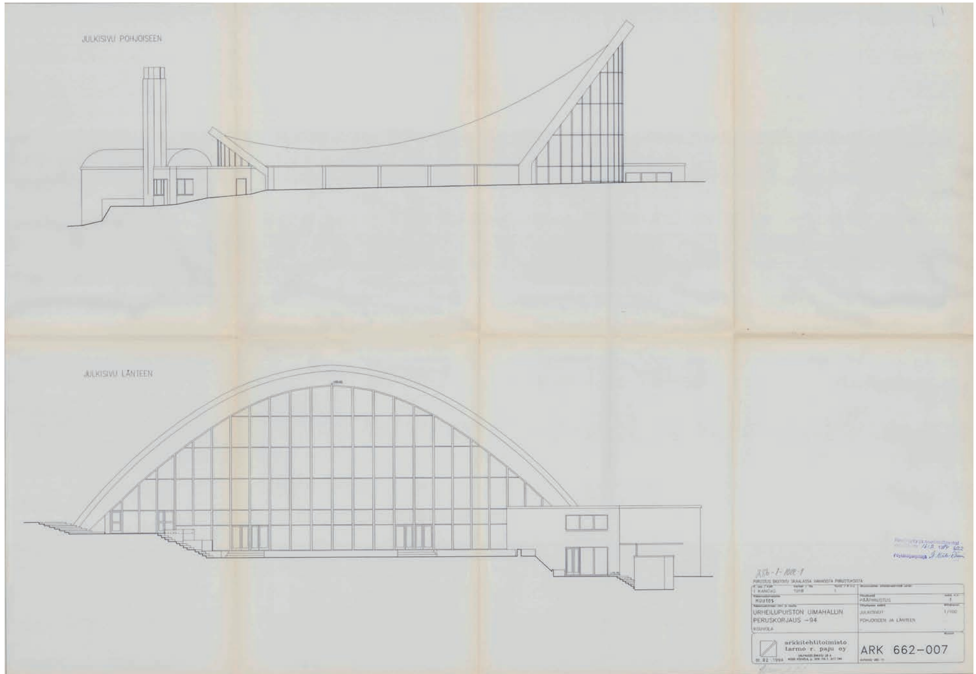
Urheilupuiston uimahallin peruskorjaus 1994. Julkisivut pohjoiseen ja länteen, päiväys 3.2.1994. Pääpiirustukset on hyväksytty 16.2.1994. Kuva: Kouvolan kaupunki, rakennusvalvonnan arkisto.
