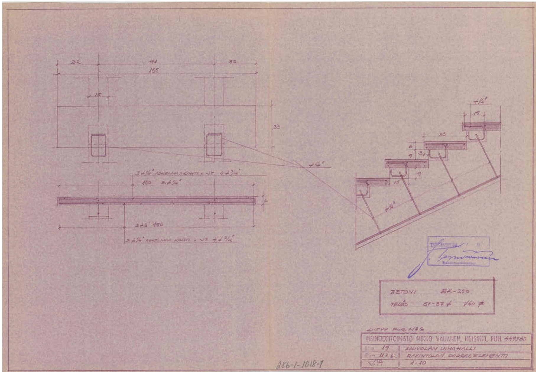
Kouvolan uimahallin ravintolan porraselementti, päiväys 11.7.1962. Rakennepiirustusnumero 19. Kuva: Kouvolan kaupunki, rakennusvalvonnan arkisto.
