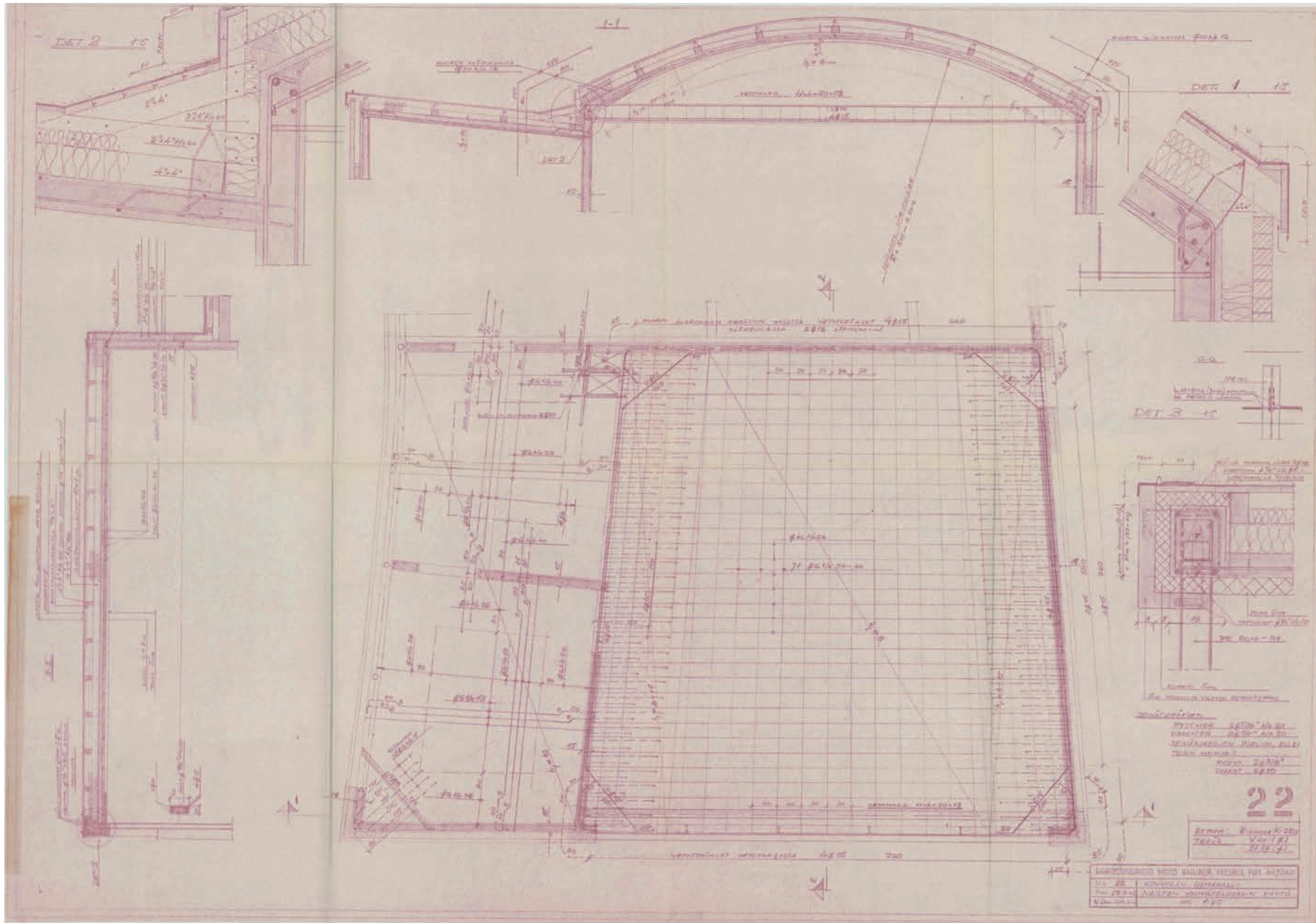
Kouvolan uimahallin naisten voimistelusalin katto, päiväys 28.9.1962. Kuvassa mm. kaarevan katon yhdistyminen lapekattoon ja räytädetaljia. Rakennepiirustusnumero 22. Kuva: Kouvolan kaupunki, rakennusvalvonnan arkisto.
