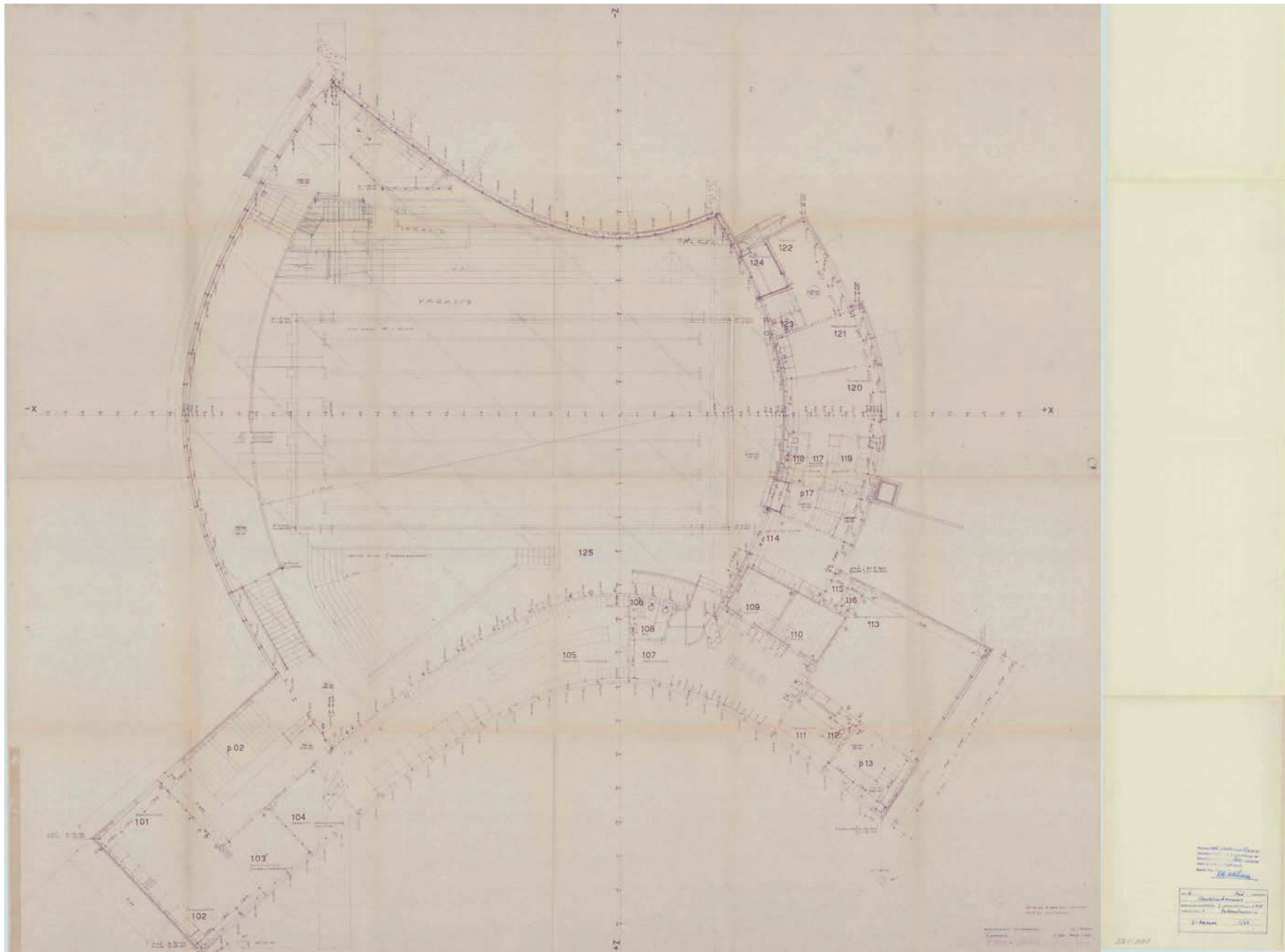
1. kerroksen pohjapiirros, päiväys 30.5.1962. Muutospäiväyksiä 14.9.1962 ja 27.10.1962. Pääpiirustukset on hyväksytty 13.12.1962 - lupaleima on kuvan taustapuolella.
