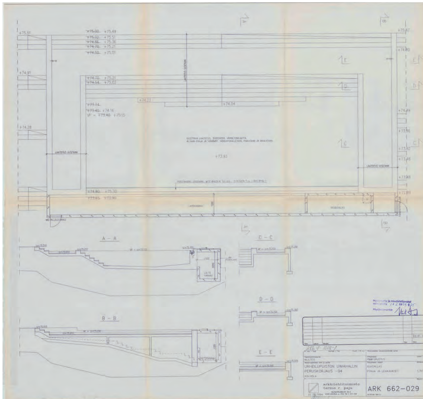
Urheilupuiston uimahallin peruskorjaus 1994. Ulkoallas pohja- ja leikkauspiirros, päiväys 31.8.1994. Uudet pääpiirustukset on hyväksytty 1.2.1995. Piirroksessa on huomioitu urakoiden aikaisia muutoksia - viimeisin muutospäiväys 2.1.1995. Kuva: Kouvolan kaupunki, rakennusvalvonnan arkisto.
