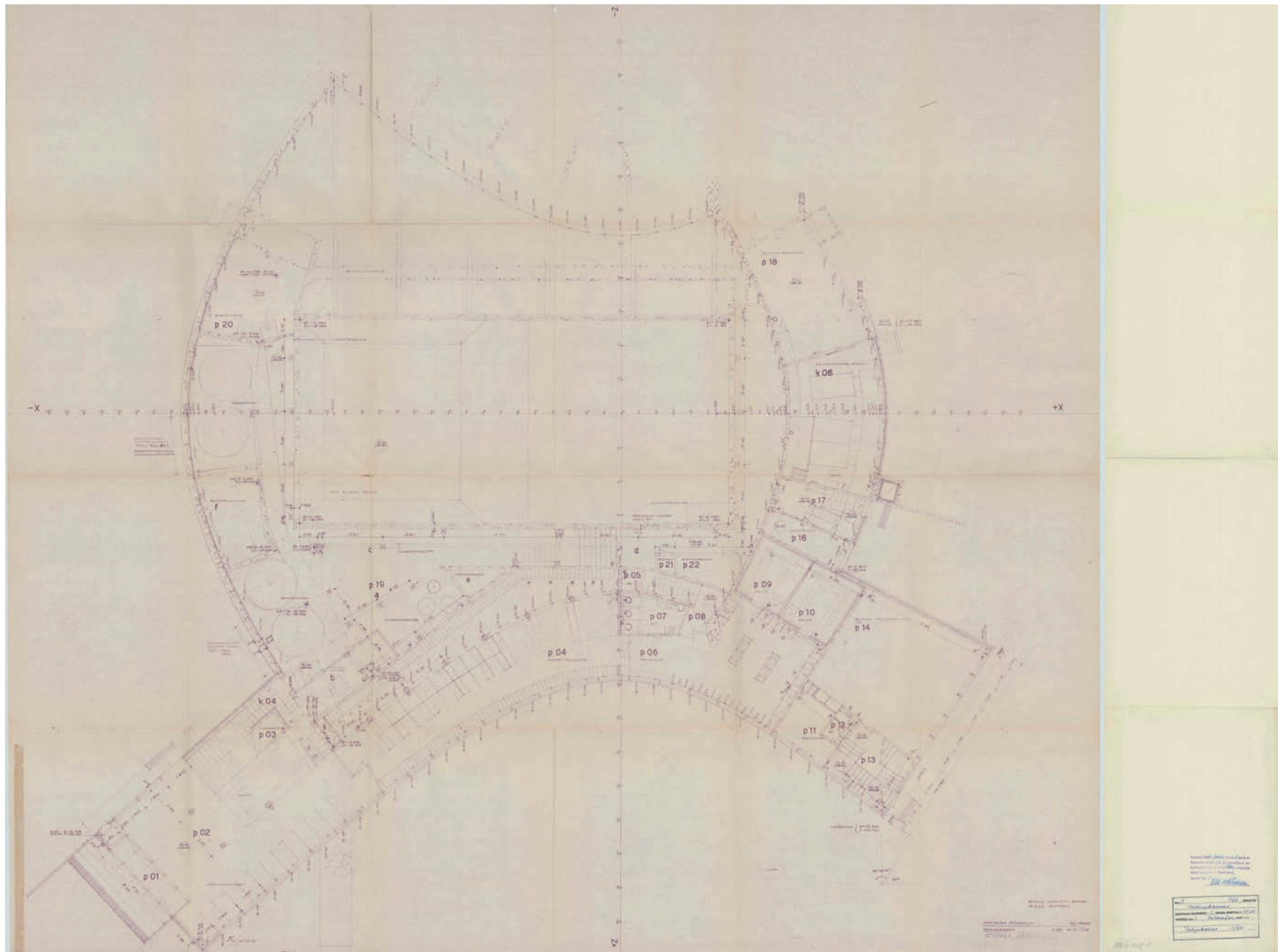
Pohjakerroksen pohjapiirros, päiväys 30.5.1962. Muutospäiväyksiä 14.9.1962 ja 27.10.1962. Pääpiirustukset on hyväksytty 13.12.1962 - lupaleima on kuvan taustapuolella.
