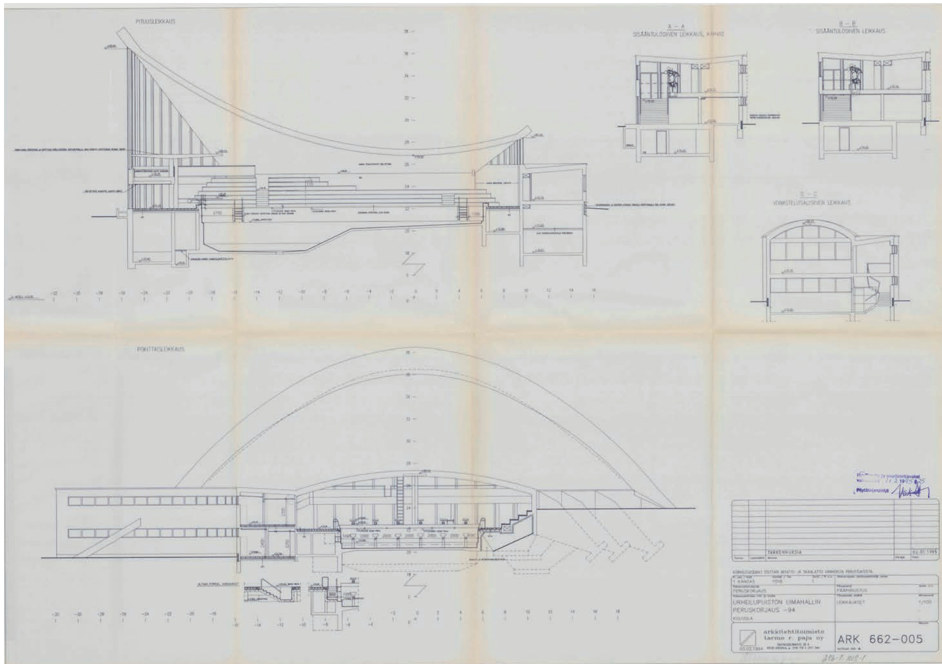
Urheilupuiston uimahallin peruskorjaus 1994. Leikkaukset, päiväys 3.2.1994. Uudet pääpiirustukset on hyväksytty 1.2.1995.
