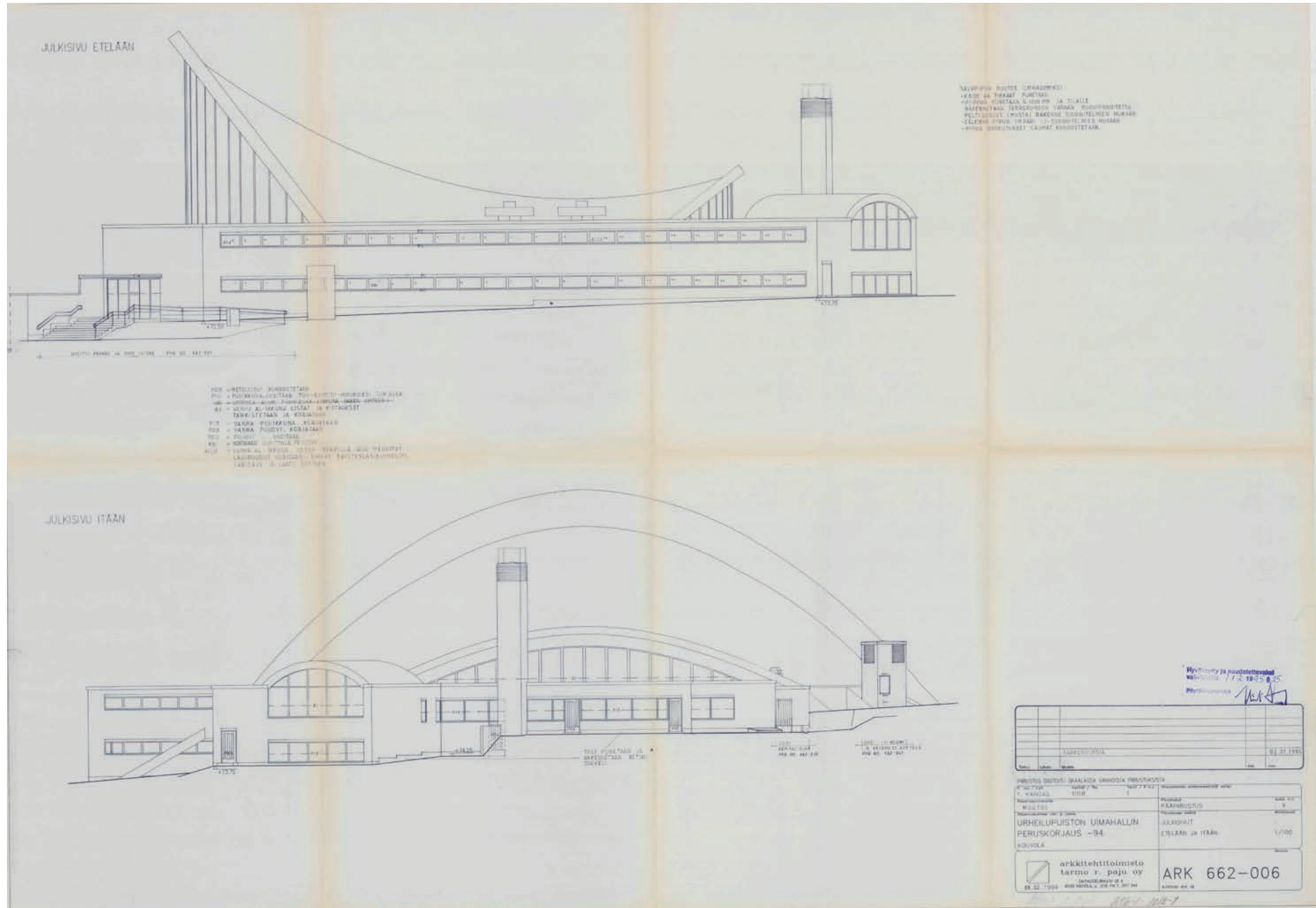
Urheilupuiston uimahallin peruskorjaus 1994. Julkisivut etelään ja itään, päiväys 3.2.1994. Uudet pääpiirustukset on hyväksytty 1.2.1995. Piirroksessa on huomioitu urakoiden aikaisia muutoksia - viimeisin muutospäiväys 2.1.1995.
