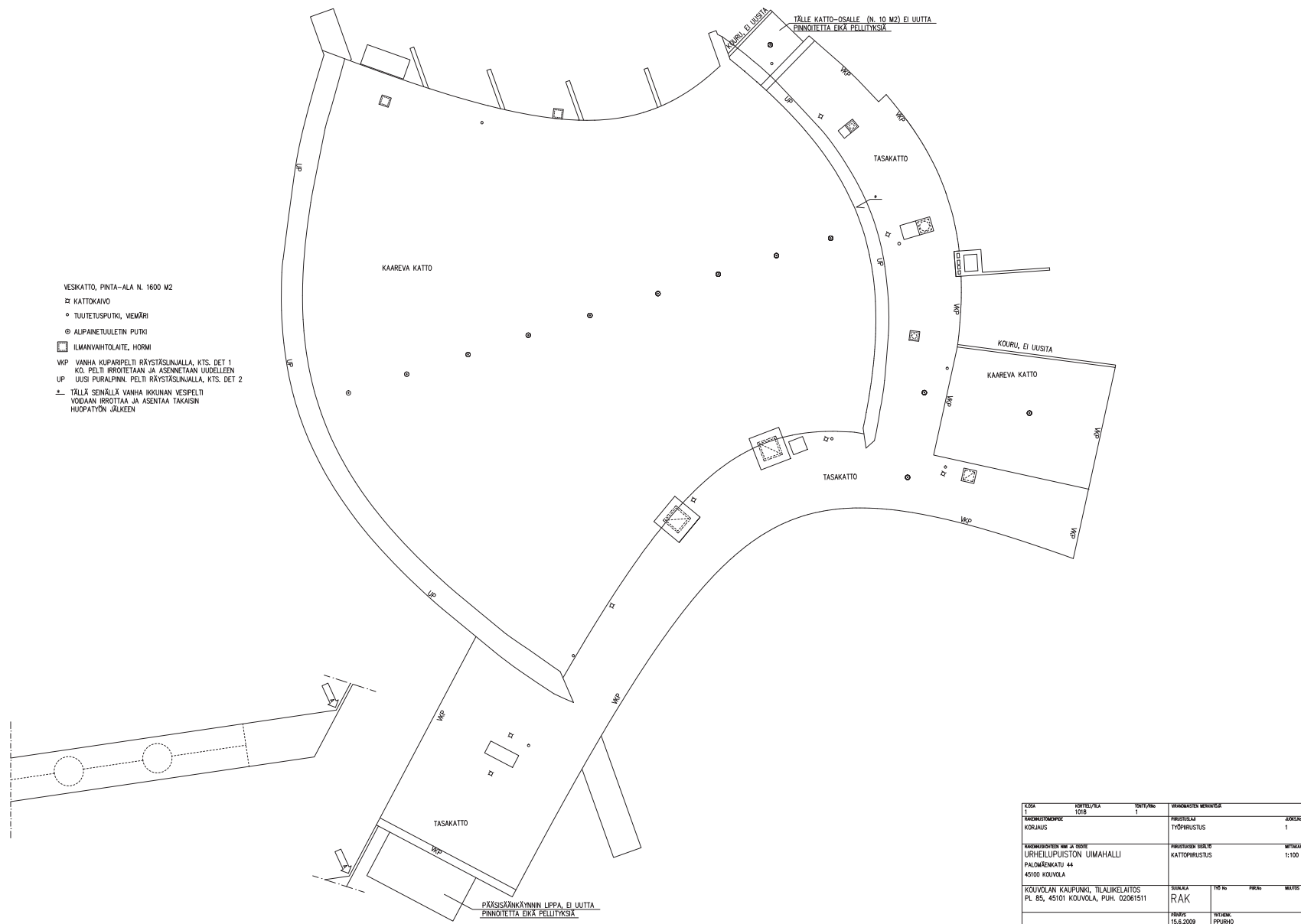
Urheilupuiston uimahallin vesikatton korjauksia, kattopiirustus, päiväys 15.6.2009.
