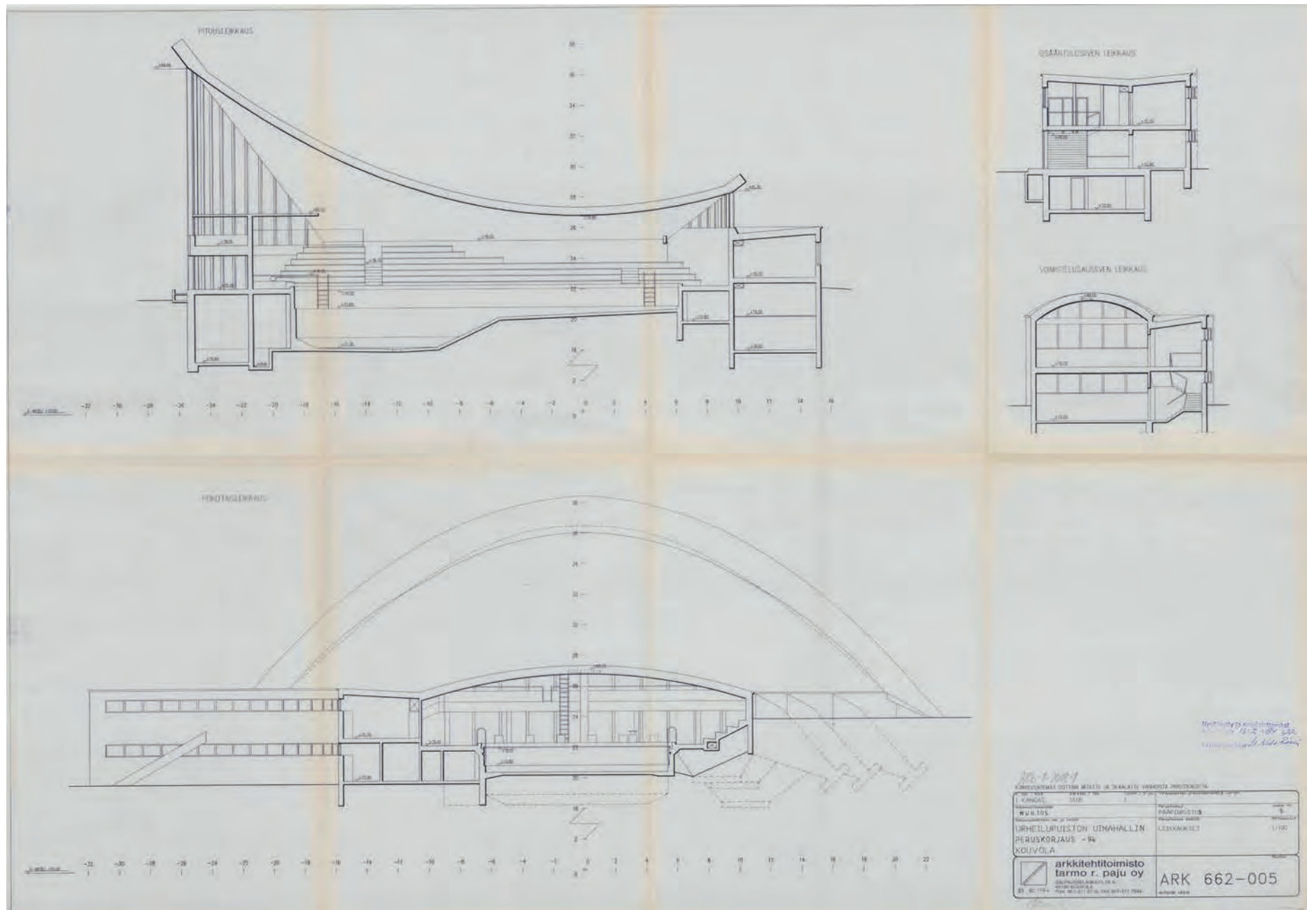
Urheilupuiston uimahallin peruskorjaus 1994. Leikkaukset, päiväys 3.2.1994. Pääpiirustukset on hyväksytty 16.2.1994. Kuva: Kouvolan kaupunki, rakennusvalvonnan arkisto.
