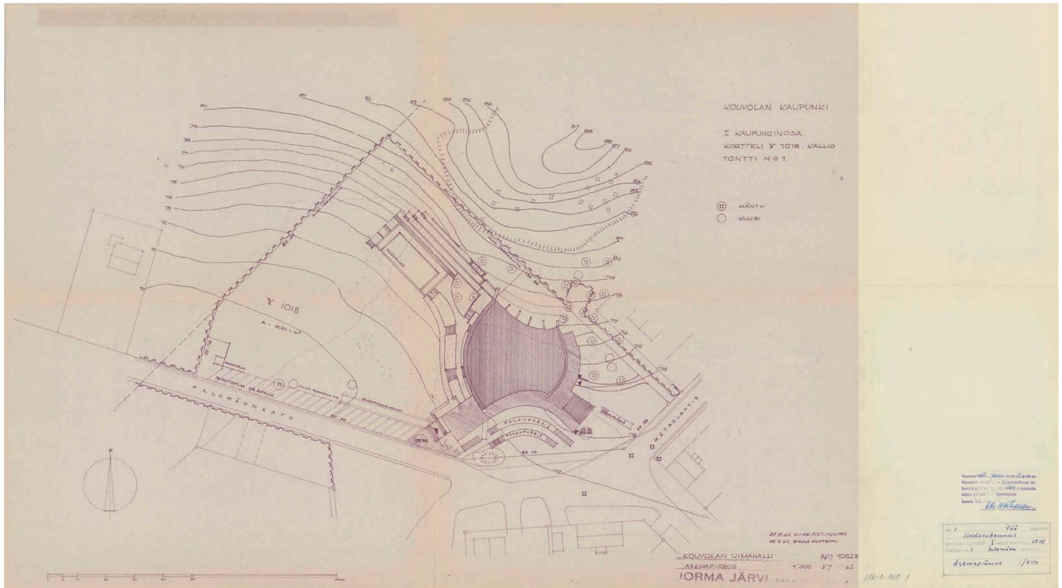
Asemapiirros, päiväys 3.7.1962. Muutospäiväyksiä 19.7.1962 ja 27.10.1962. Pääpiirustukset on hyväksytty 13.12.1962 - lupaleima on kuvan taustapuolella. Kuva: Kouvolan kaupunki, rakennusvalvonnan arkisto.
