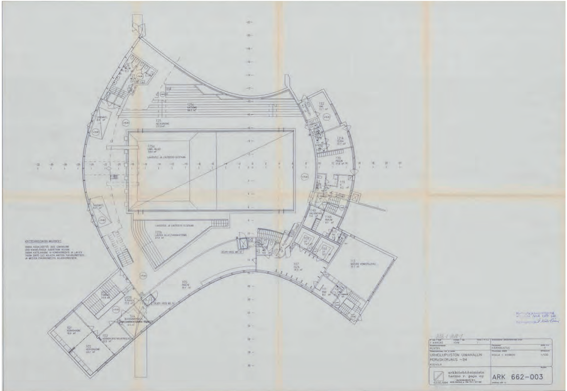
Urheilupuiston uimahallin peruskorjaus 1994. Pohjapiirros, 1. kerros, päiväys 3.2.1994. Pääpiirustukset on hyväksytty 16.2.1994. Kuva: Kouvolan kaupunki, rakennusvalvonnan arkisto.
