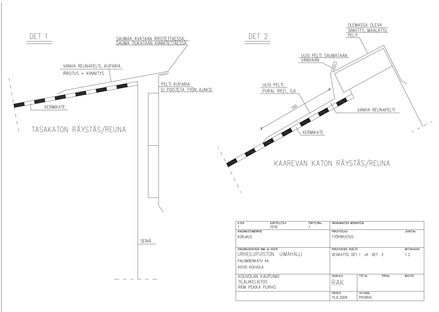
Urheilupuiston uimahallin vesikaton korjauksia, vesikatto detaljia, päiväys 15.6.2009. Kuva: Kouvolan kaupunki, Konsernipalvelut, Tilapalvelut.
