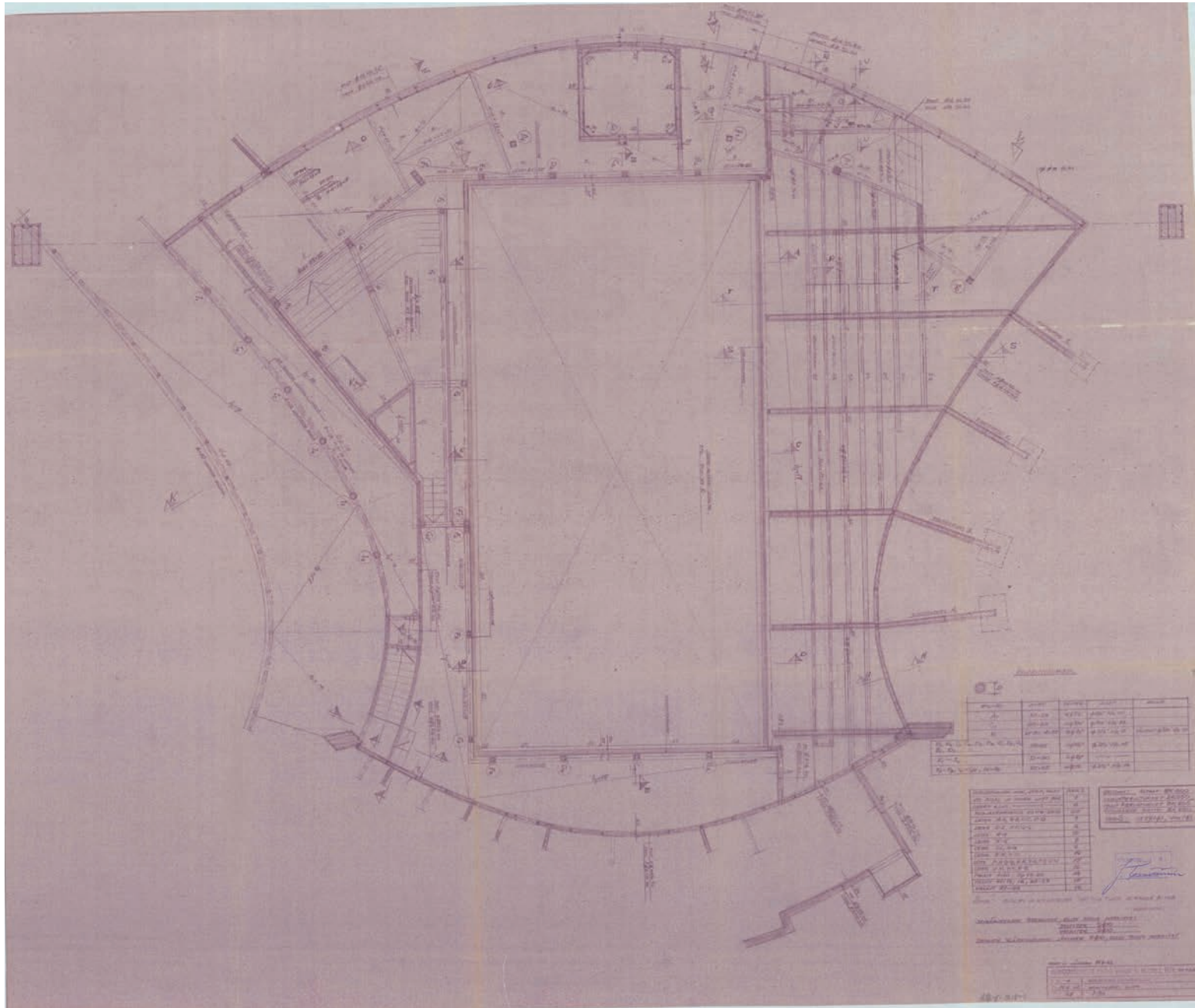
Kouvolan uimahallin pohjakerroksen katto, päiväys 7.6.1962. Kuvassa on mm. kontreforien (tukipilarien) asemat numeroitu. Jokaisesta tukipilarista on omat rakennekuvat. Rakennepiirustusnumero 4. Kuva: Kouvolan kaupunki, rakennusvalvonnan arkisto.
