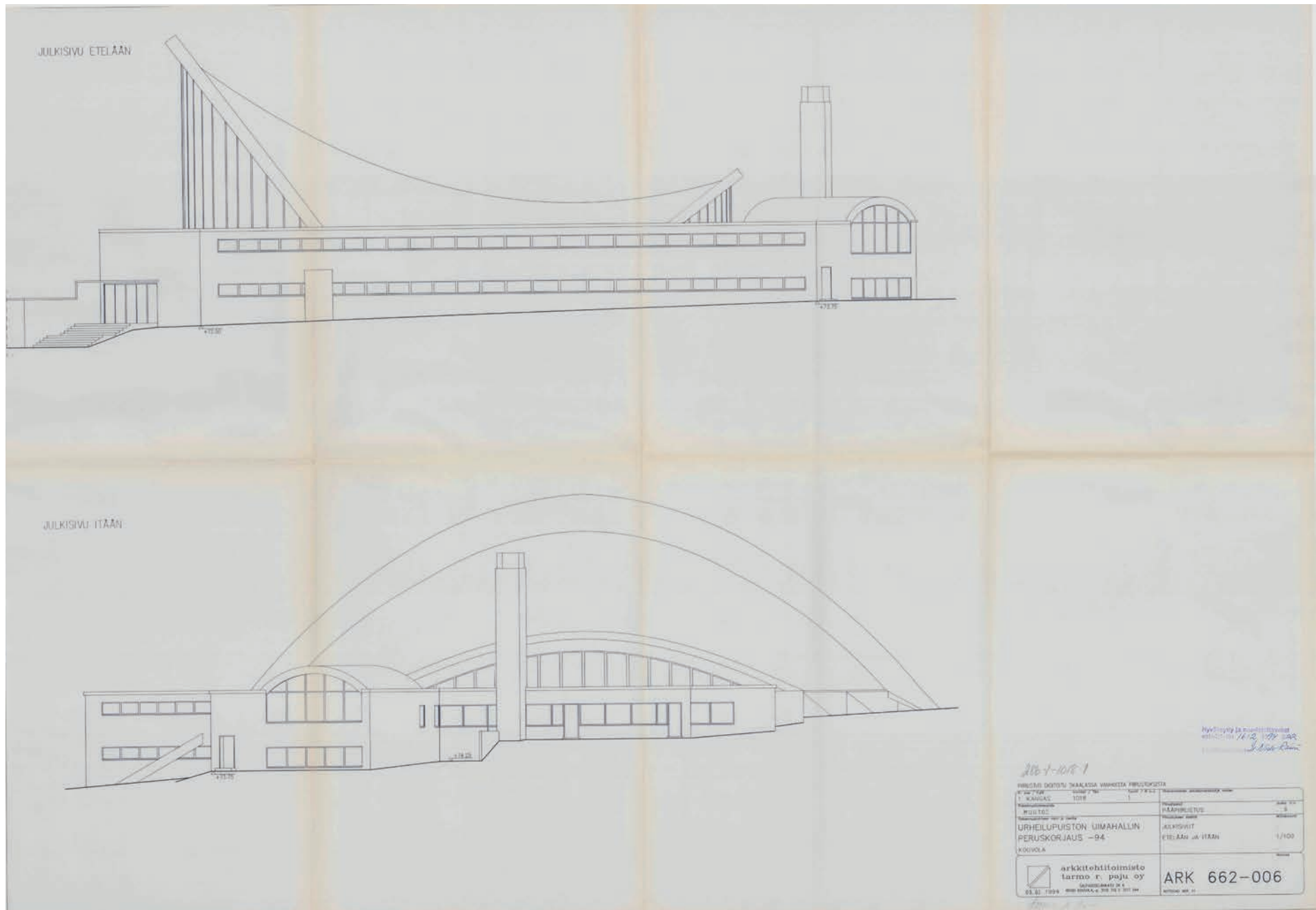
Urheilupuiston uimahallin peruskorjaus 1994. Julkisivut etelään ja itään, päiväys 3.2.1994. Pääpiirustukset on hyväksytty 16.2.1994. Kuva: Kouvolan kaupunki, rakennusvalvonnan arkisto.
