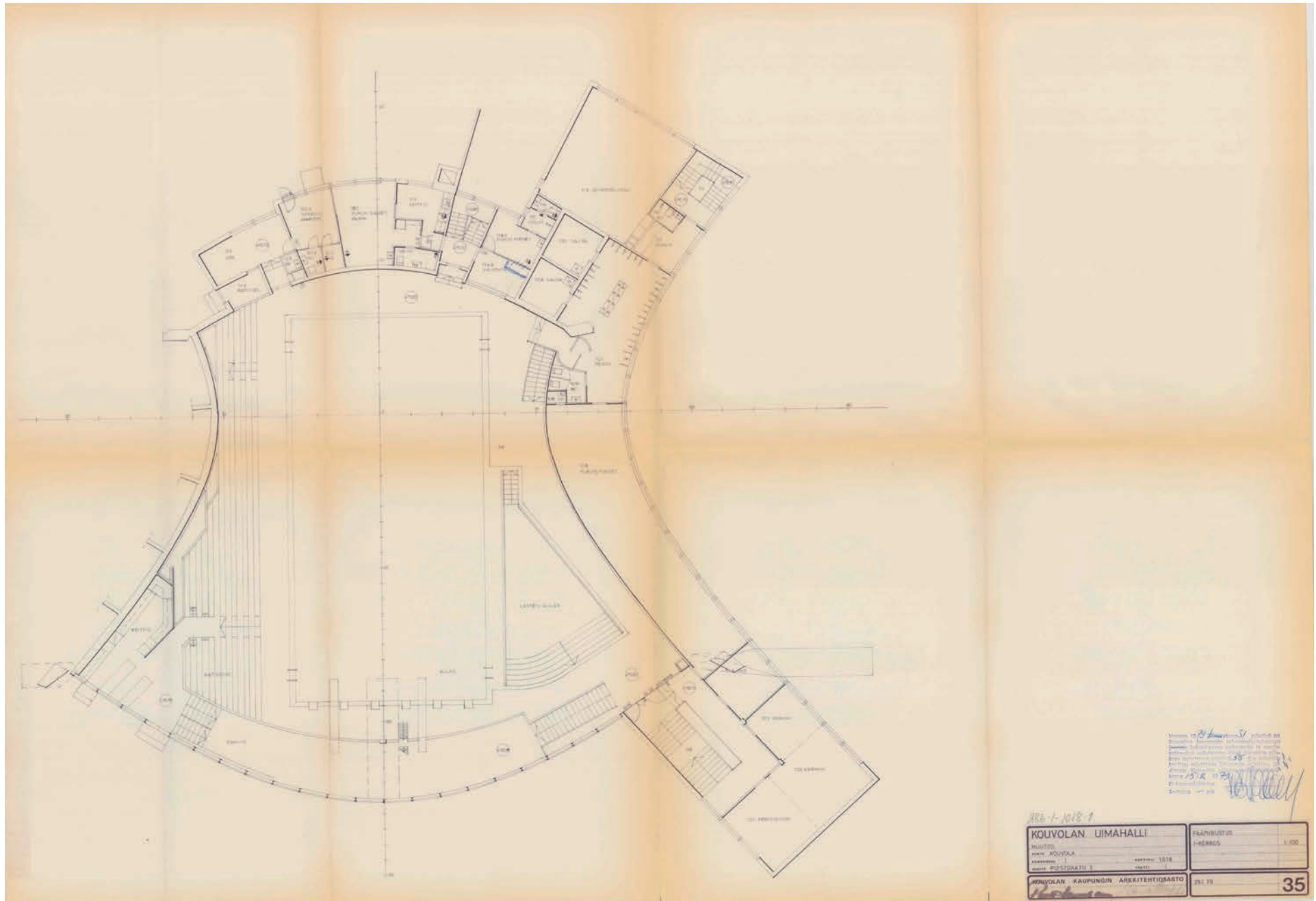
Kouvolan uimahallin talonmiehen asunnon muutos sosiaalitiloiksi ja sisääntuloalaan johtavien ovien sekä lasiseinän muutos, päiväys 22.1.1979. Pääpiirustukset on hyväksytty 31.1.1979.
