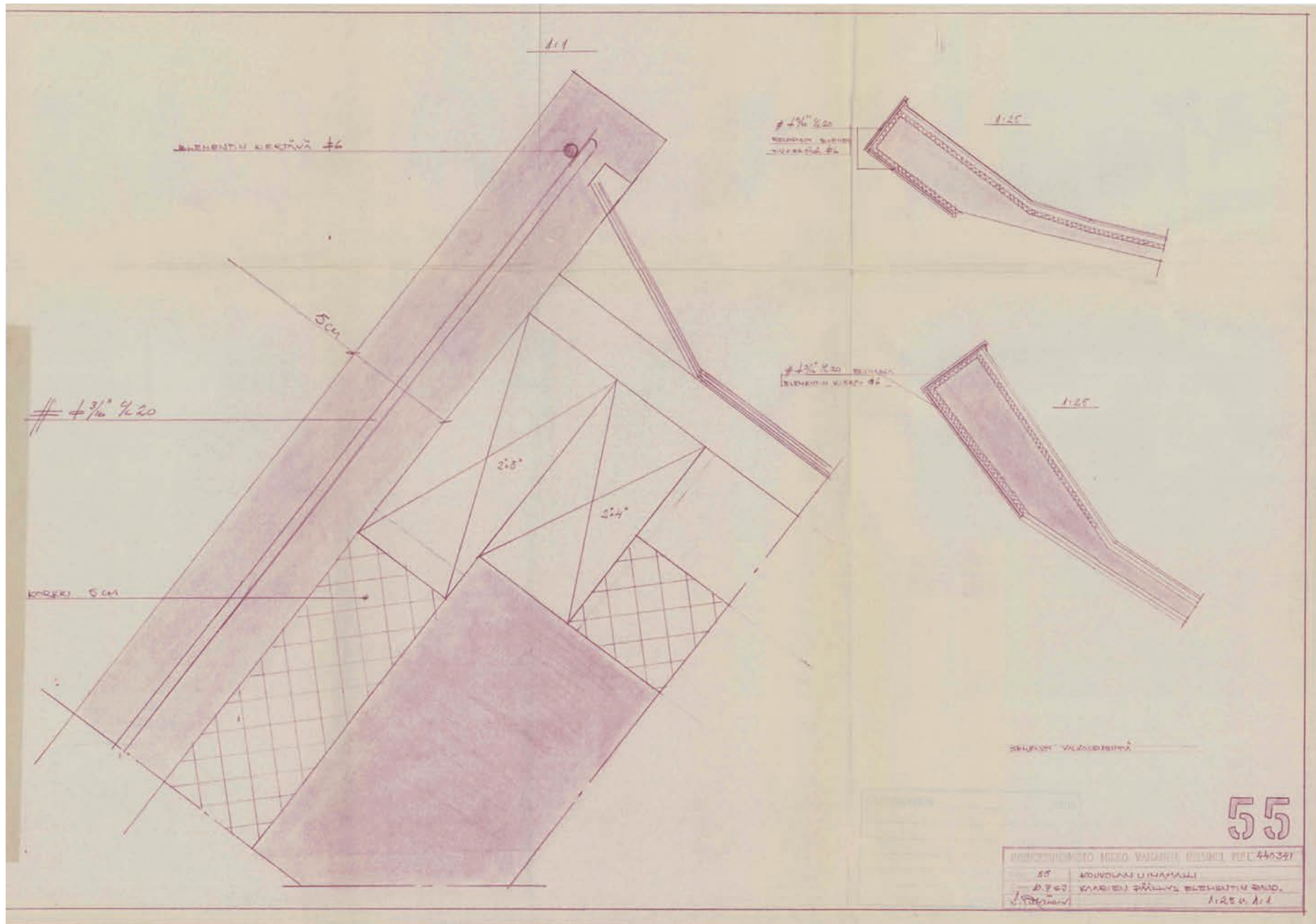
Kouvolan uimahallin kaarien päällys elementtien rauditus, päiväys 10.7.1963. Rakennepiirustusnumero 55.
