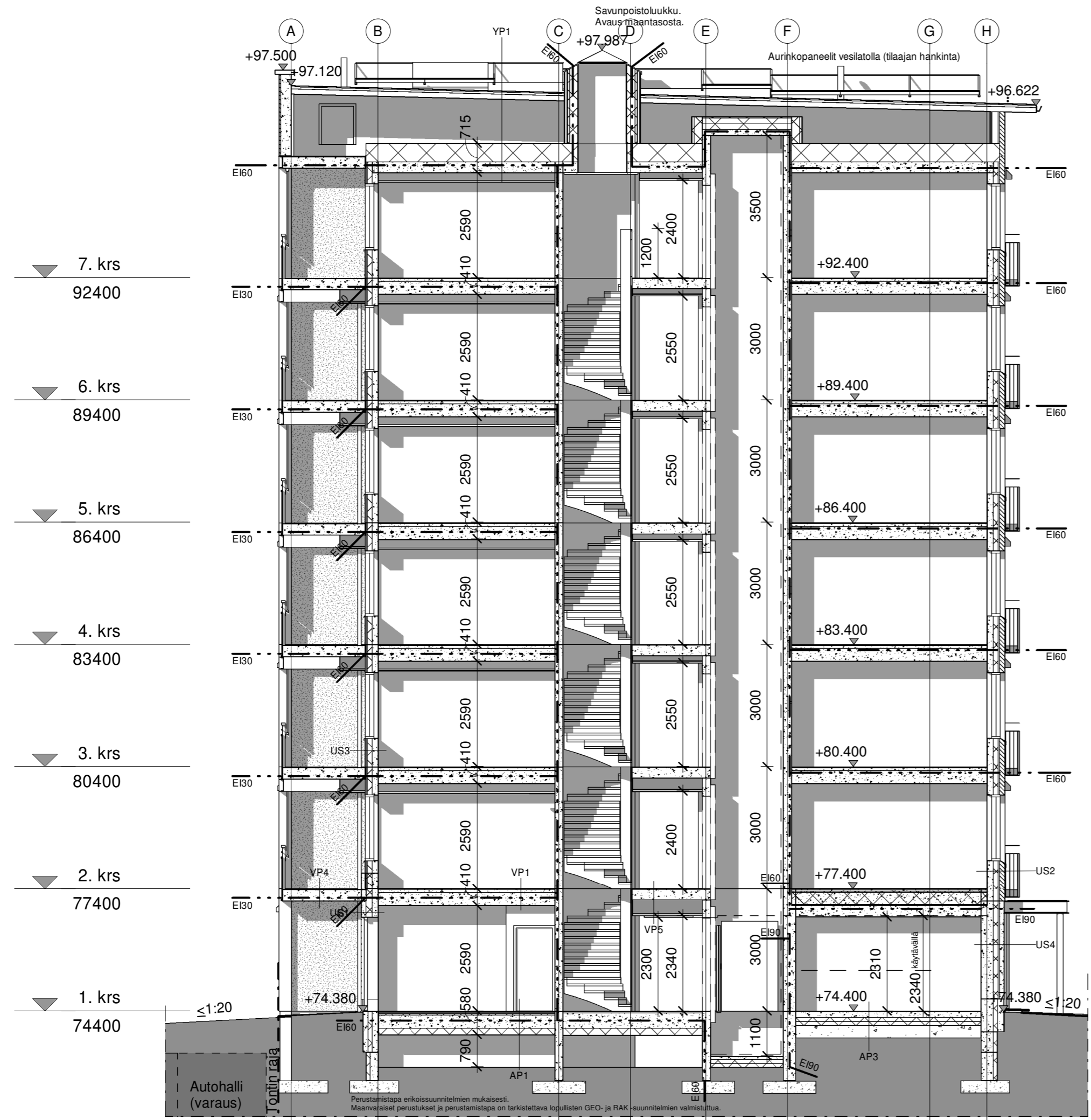
Leikkaus A-A, 1:100
